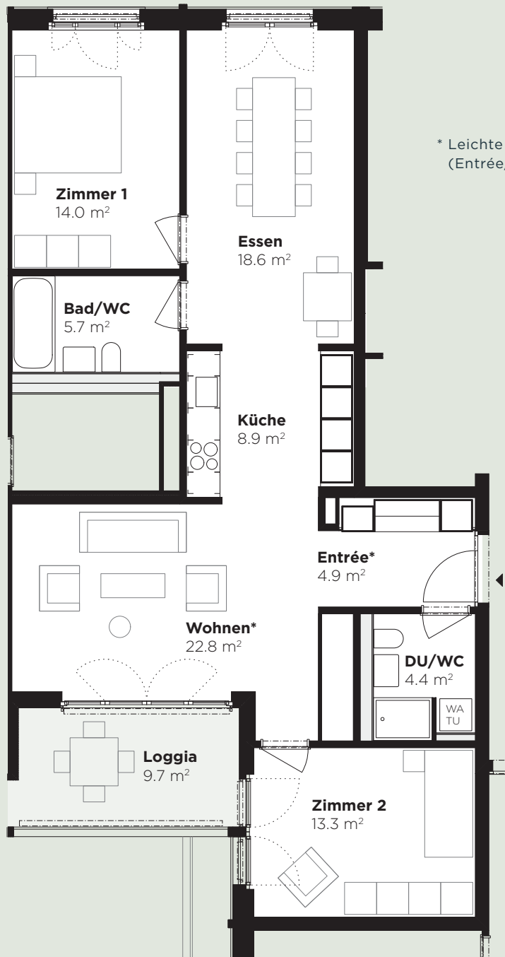
Abbildung: 2. Obergeschoss, Wohnung 86.214
