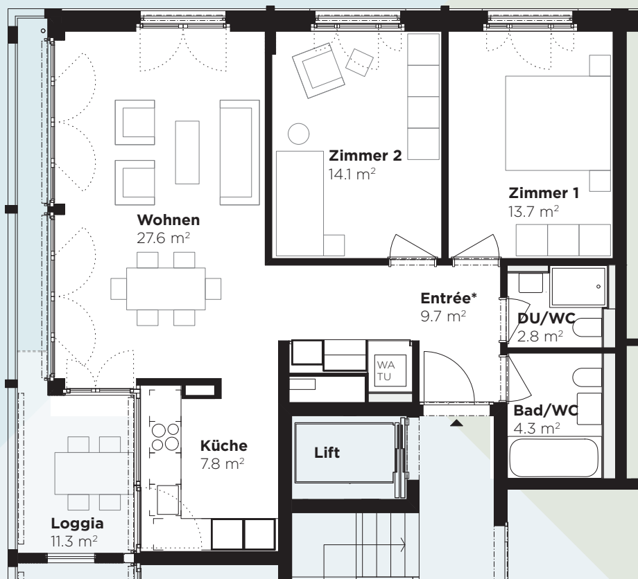
Abbildung: 2. Obergeschoss, Wohnung 82.207
